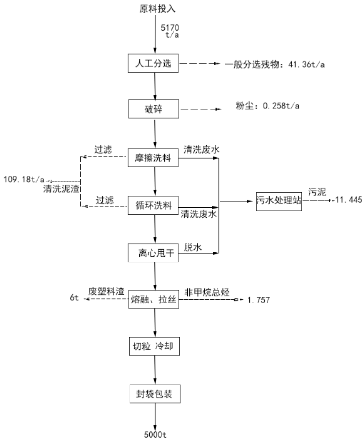
图 2.3-3项目物料平衡图 (单位: t/a)
