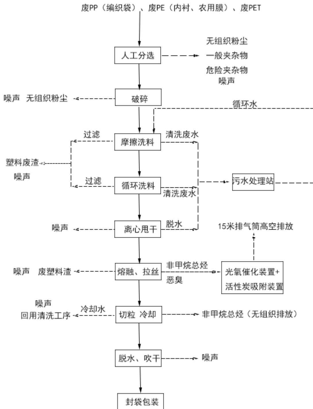
图 2.3-2 项目运营期产污环节图
