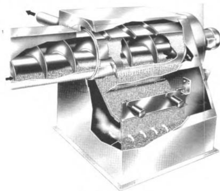
图 22-4 丸尘分离器示意图
